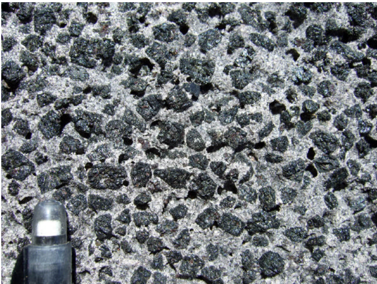
単斜輝石の大型斑晶 (~1cm) が濃集した極めて珍しい玄武岩 (写真 中野俊)
