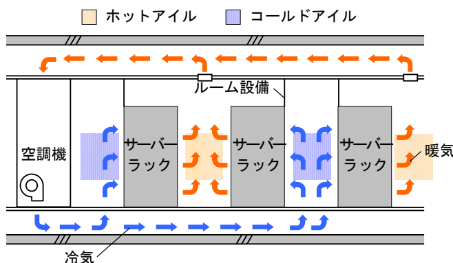
ルーム設備、ラック設備の導入例
