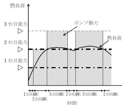
チューニング前の運転状況
