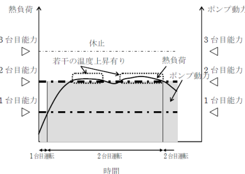
チューニング後の運転状況
