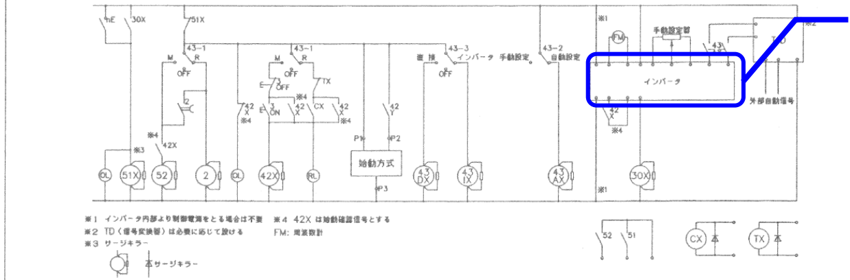
15-2 可変速運転 (バイパス回路付)
