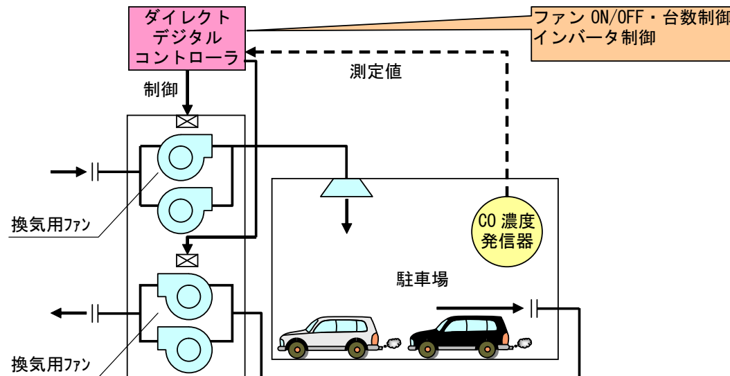
駐車場ファンのCO濃度制御
