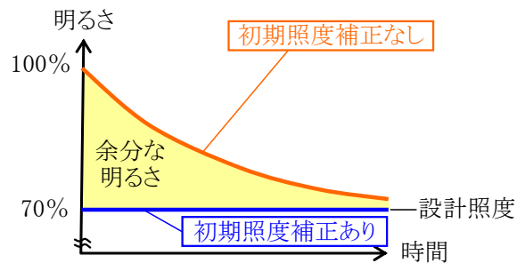
初期照度補正制御による効果
