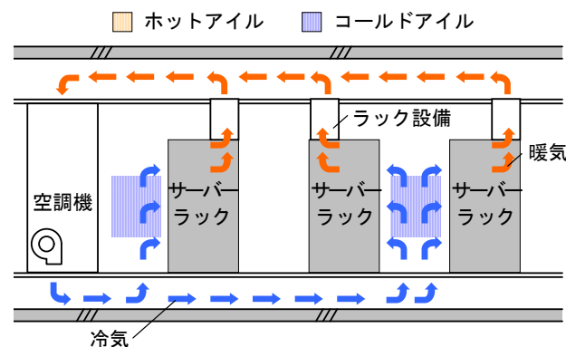
ルーム設備、ラック設備の導入例
