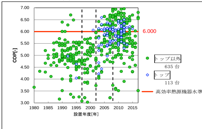
図1 ターボ冷凍機の設置年度別の機器COP分布
