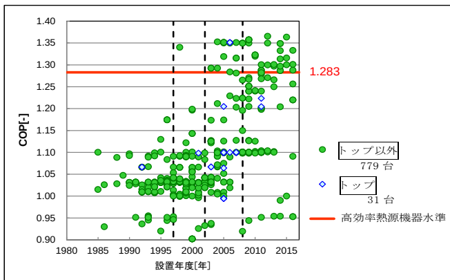
図2 直焚吸収冷温水機の設置年度別の機器COP分布
