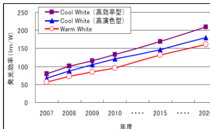
図4 LEDの発光効率のロードマップ
