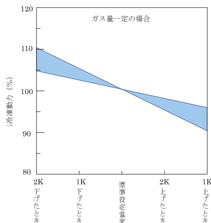
冷却水入口温度を変化させた場合の冷凍能力の変化 (ガス焚冷凍温水発生機)
