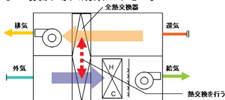
全熱交換器の採用例
