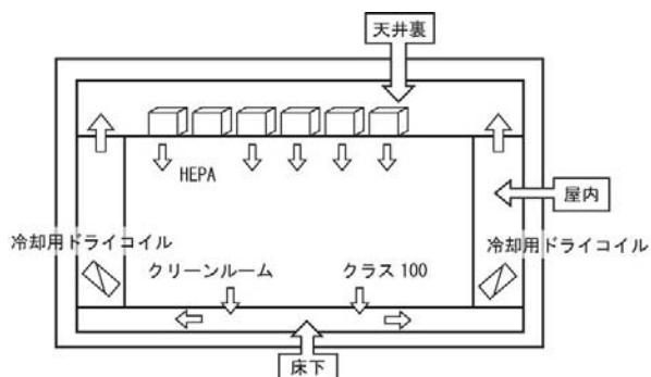
ファンフィルタユニット
