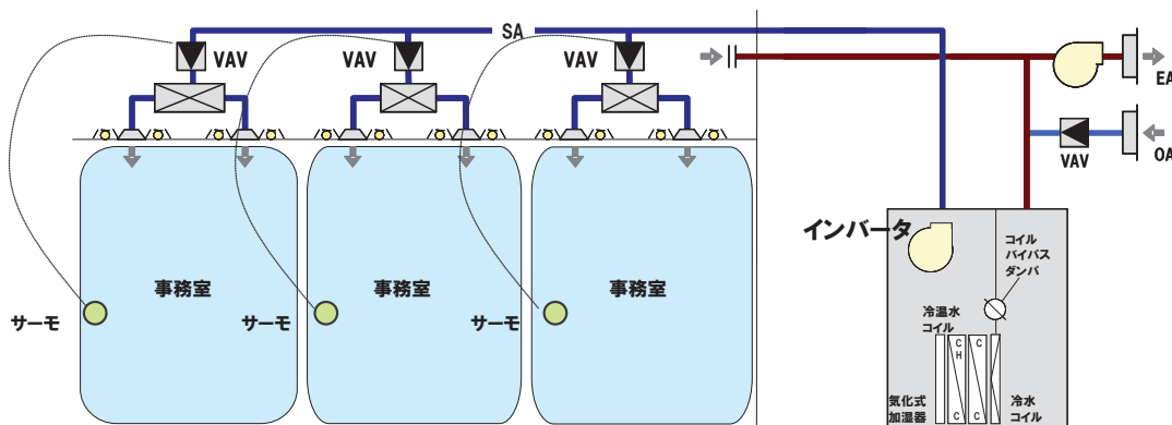
変風量システムの例
