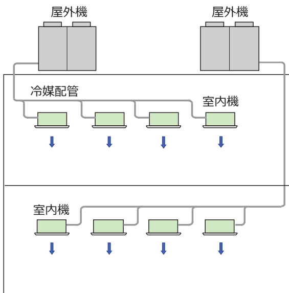
パッケージ形空調機
