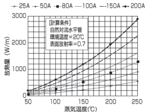
非保温蒸気管からの放熱量
