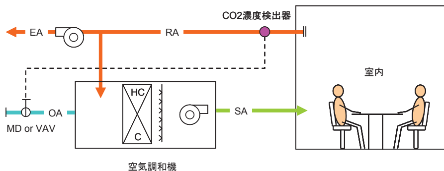
空気調和機 空調機廻りの制御フローの例
