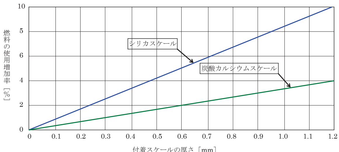
スケール付着と燃料増加率
