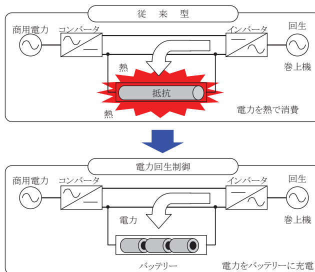
電力回生制御イメージ図
