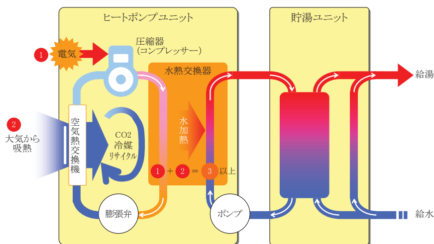
自然冷媒ヒートポンプ給湯器
