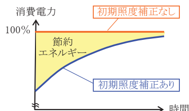
初期照度補正制御による効果
