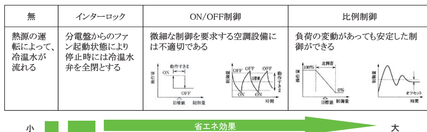
ファンコイルユニットのバルブ制御方法
