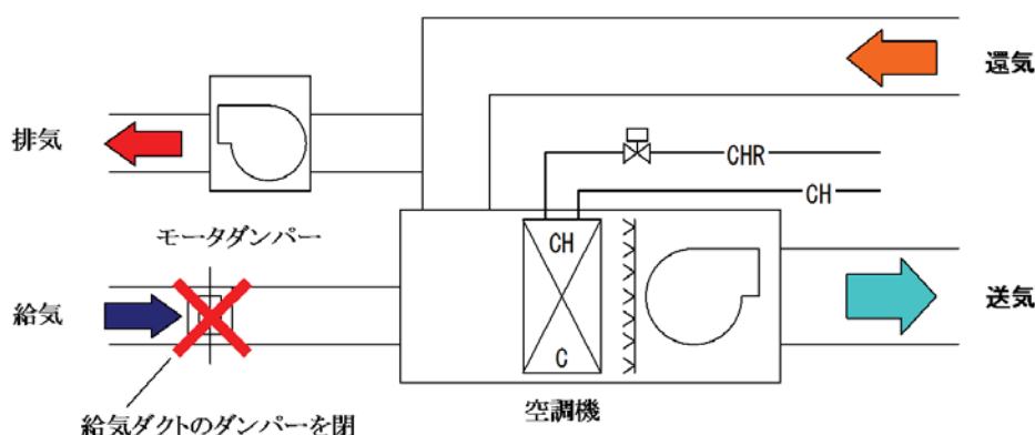
外気遮断時のイメージ
