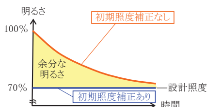
初期照度補正制御による効果
