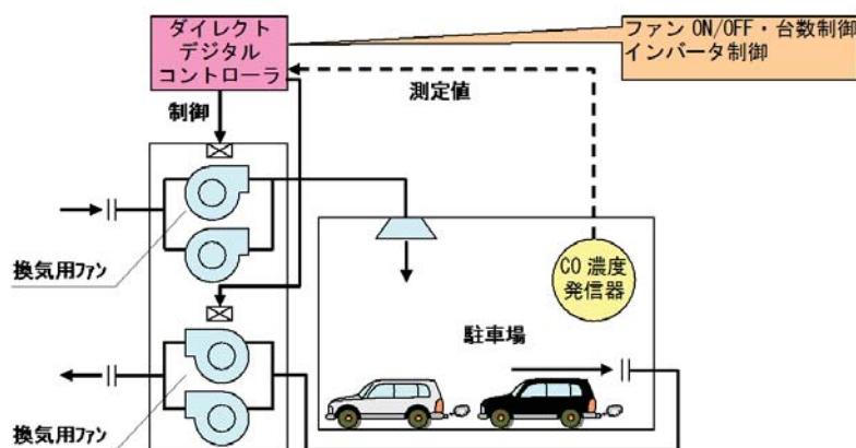
駐車場ファンのCO濃度制御
