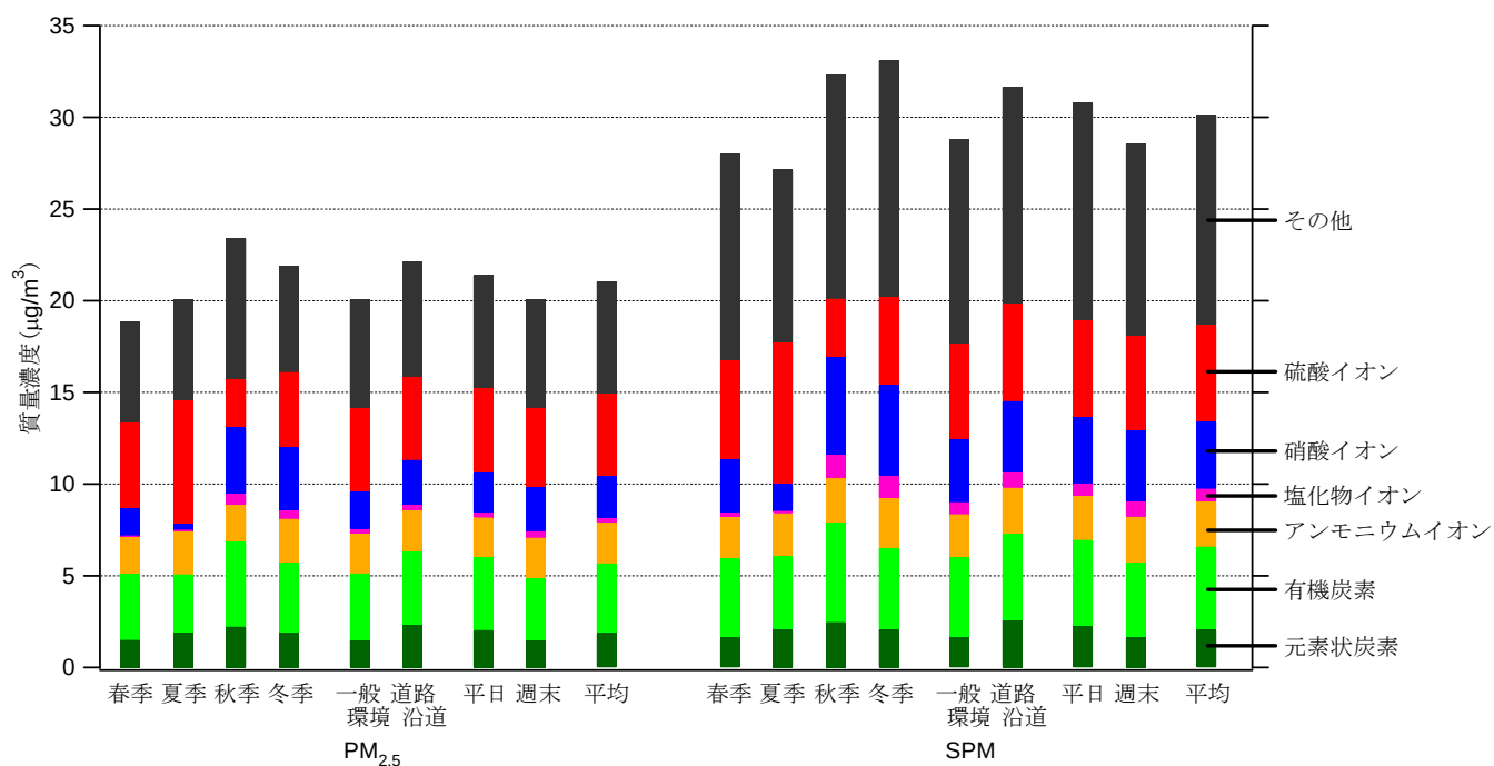
図1 大気環境調査結果（成分濃度は主要な6成分のみを示した）
