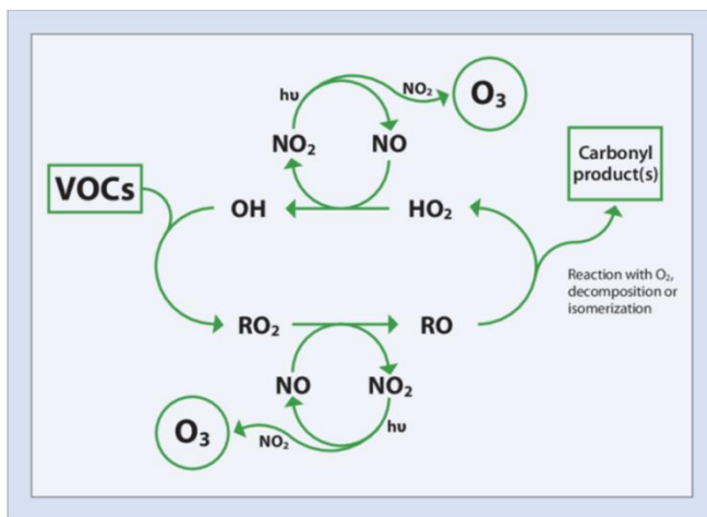
図 3-55 光化学オキシダントの生成メカニズム概要図（WHO EUOPE (2008) より引用 24,25 ）
