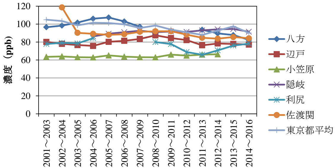
図 2-21 島しょ部等における年間4番目に高い日最高8時間値の3年移動平均の推移（光化学オキシダント）
