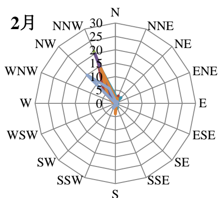
図 1-14 風配図 (10月から3月)
