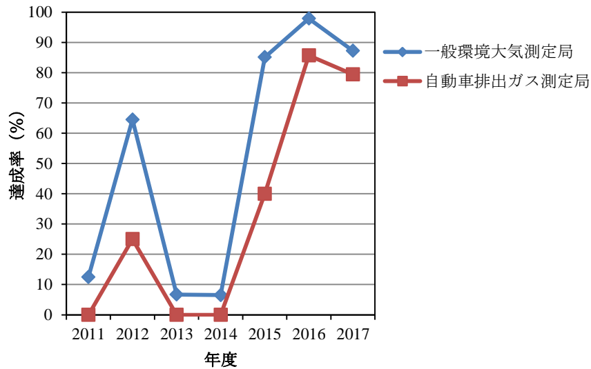
図 1-2 PM 2.5 環境基準の達成率
