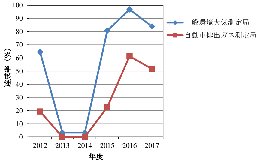
図 1-4 継続測定局における PM 2.5 環境基準の達成
