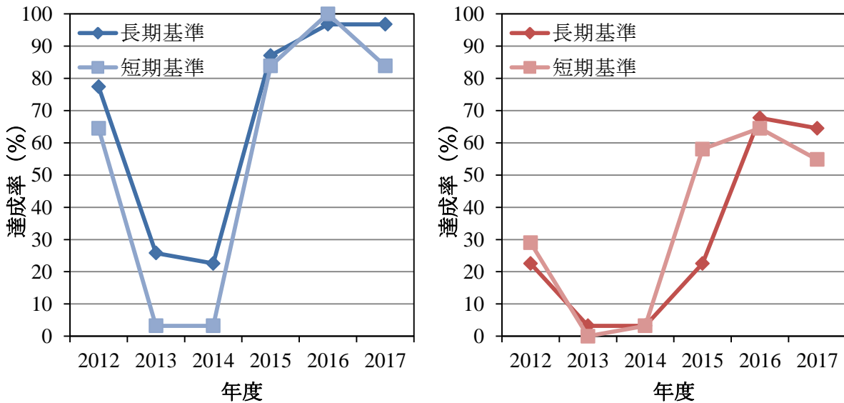
図 1-5 継続測定局における長期基準、短期基準の達成率
