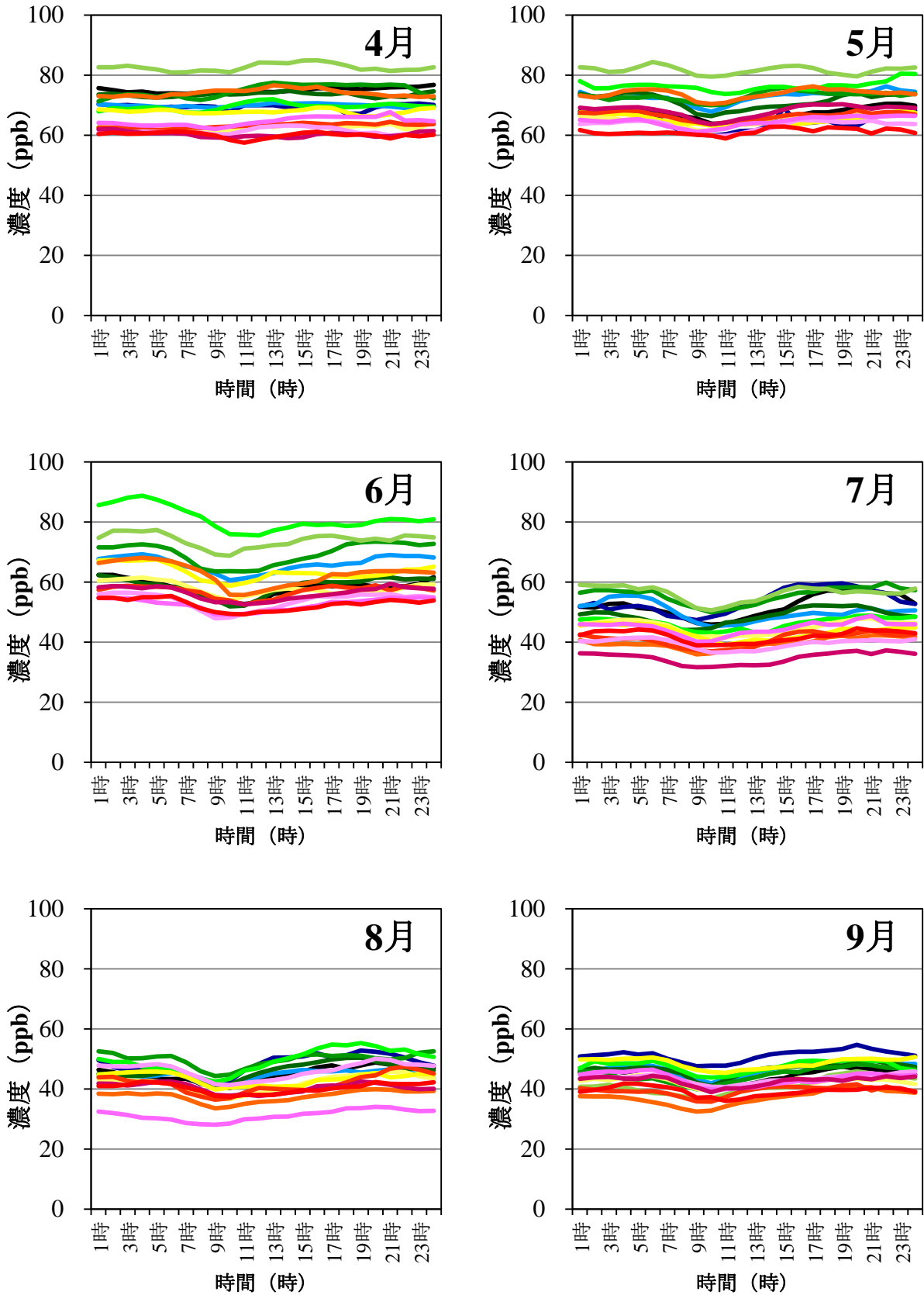
参考図 3 島しょ部等における Ox 日内変動 (4-9 月) 八方尾根
