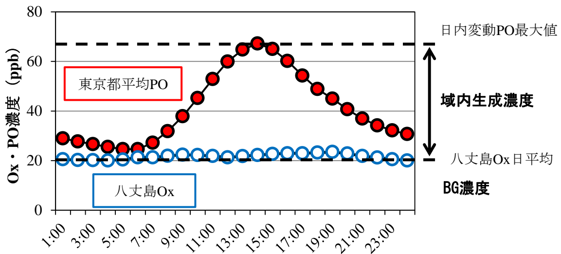
図 2-26 都内光化学オキシダントのバックグラウンド（BG）濃度、域内生成濃度の算出イメージ
