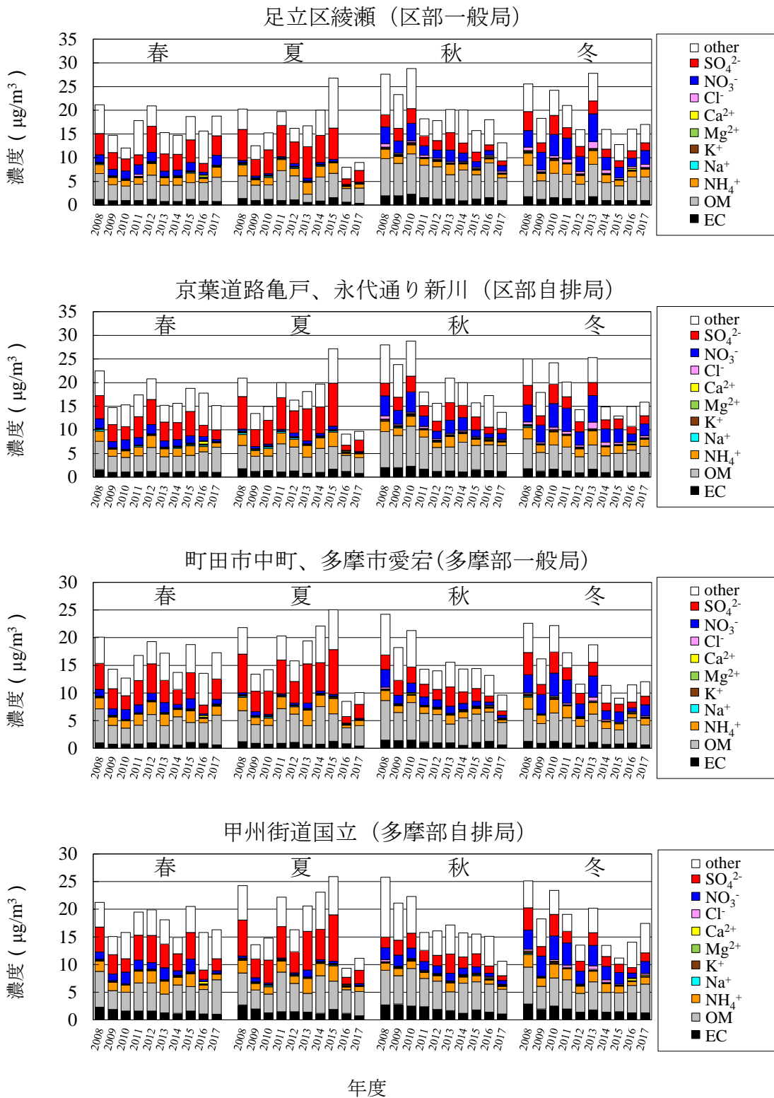
図 1-16 各季節の PM 2.5 成分濃度の経年変化
