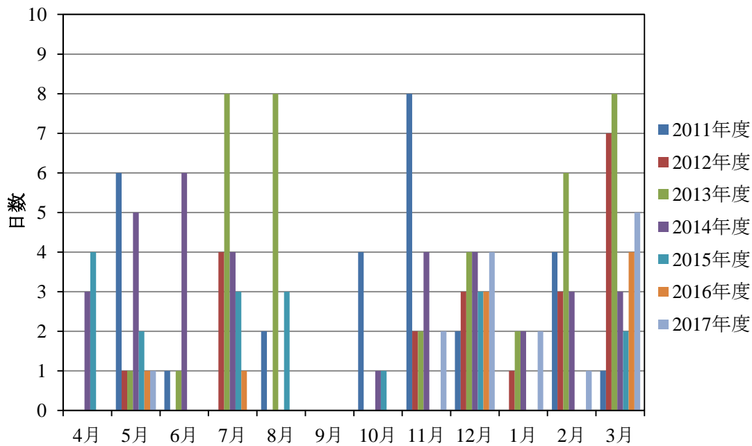
図 1-6 東京都内一般環境大気測定局の PM 2.5 日平均値が 35 µg/m 3 を超過した日数
