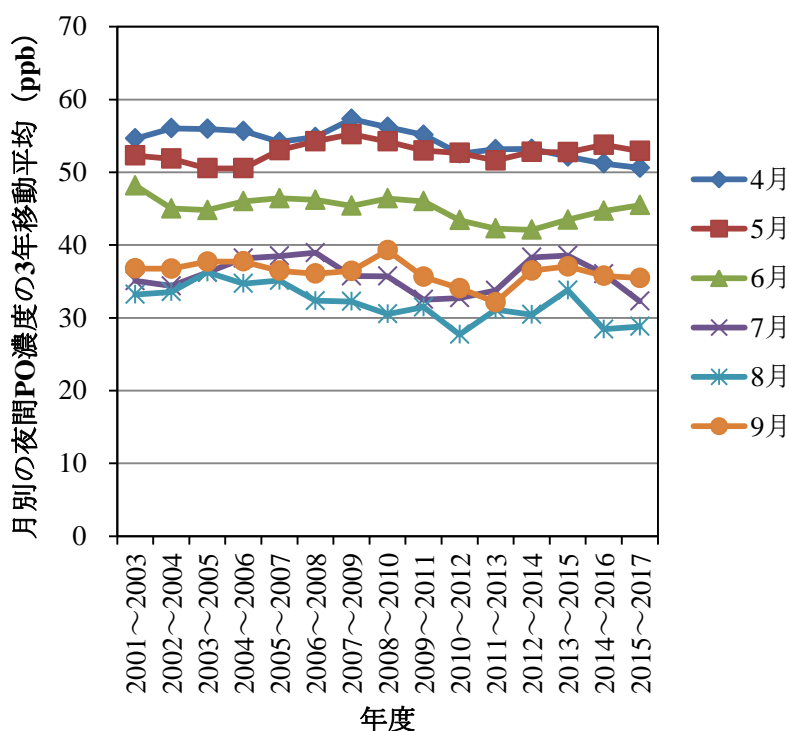
図 2-11 暖候期における月別の夜間ポテンシャルオゾン (PO) 濃度の 3 年移動平均の推移
